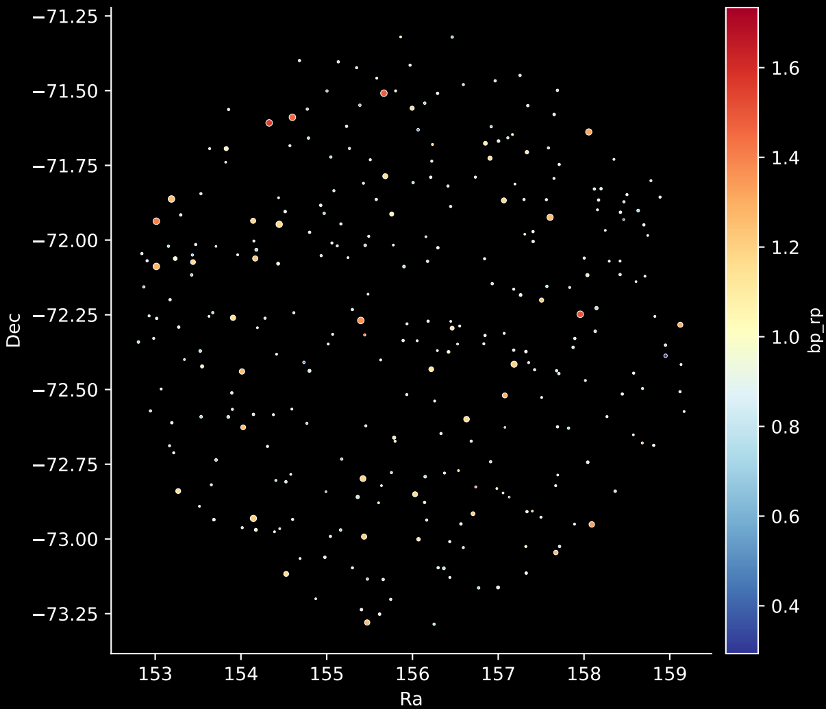
GALAH DR4 Field: [259] Stars: 298
