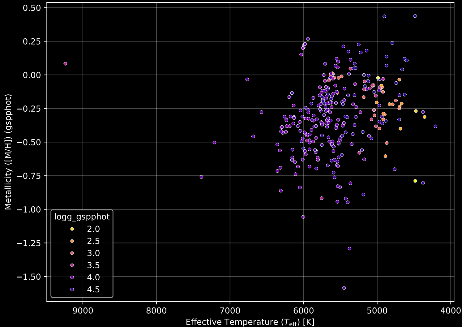
GALAH DR4 Field: [259] Stellar Population Parameters (n= 298)
